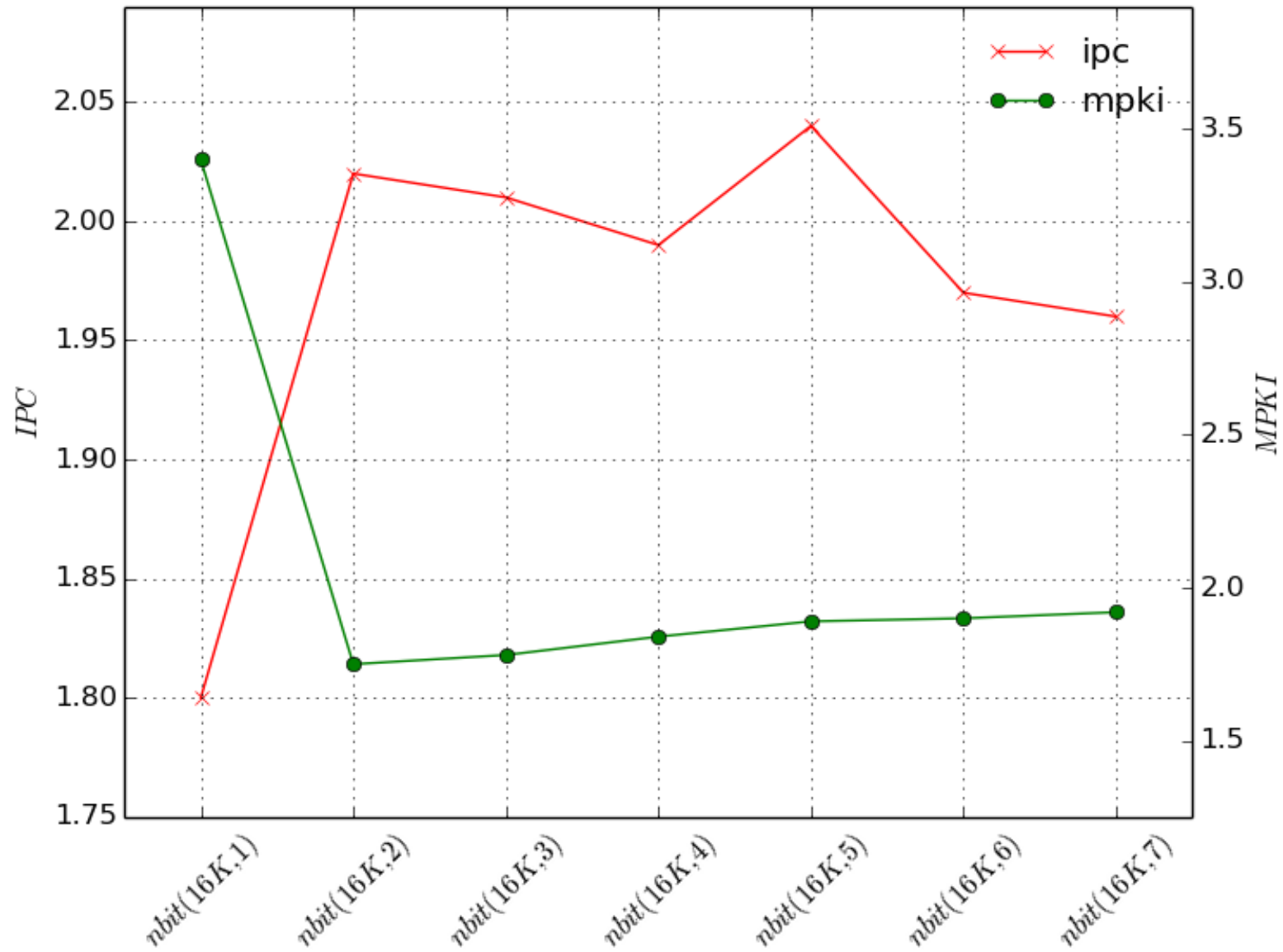
IPC vs MPKI
